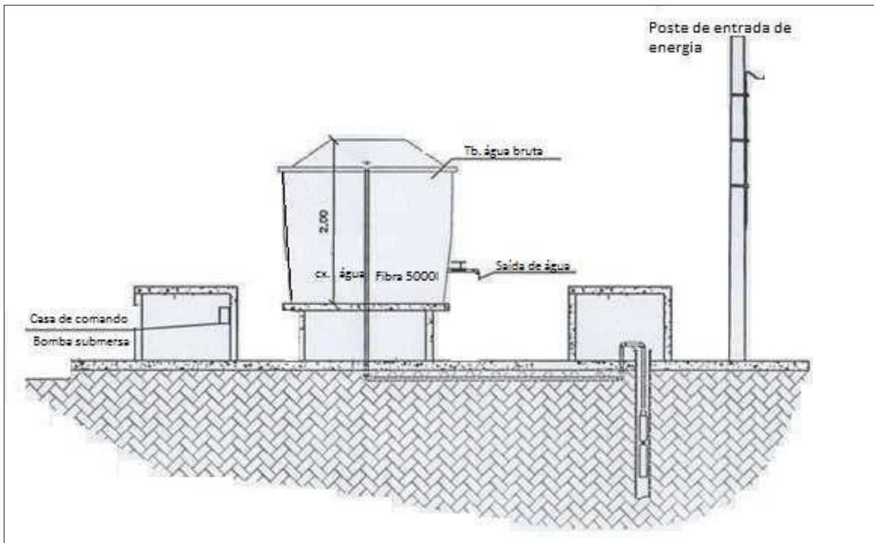
SISTEMA DE DESSALINIZAÇÃO DE AGUA – S.D.A (PLANTA BAIXA E CORTE – ABRIGO E MURO DE ALVENARIA)
