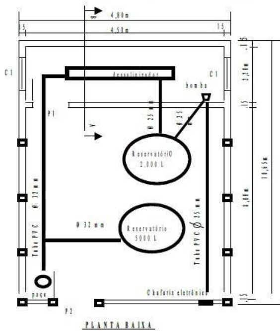
SISTEMA DE DESSALINIZAÇÃO DE AGUA – S.D.A (PLANTA BAIXA E CORTE – ABRIGO E MURO DE ALVENARIA)
